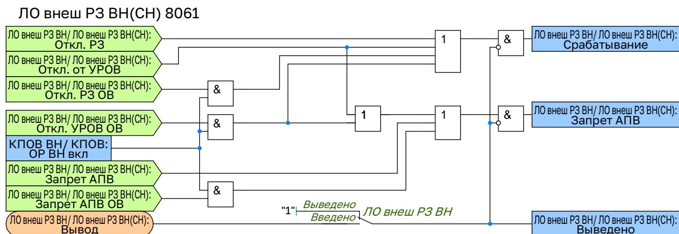
Рисунок 2.36 – Функциональная схема логики внешних отключений ВН
