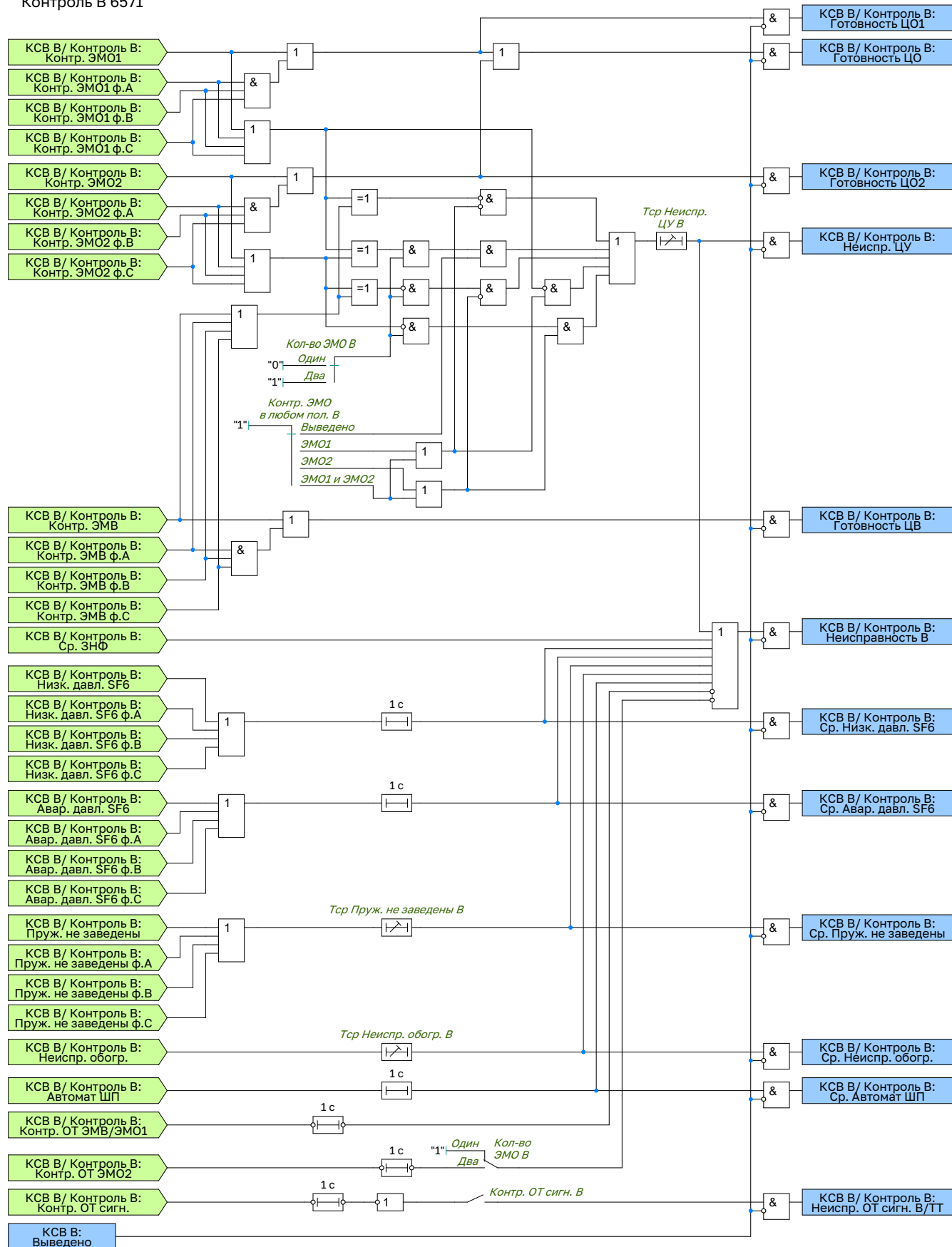
Рисунок 2.31 – Функциональная схема логики контроля выключателя
