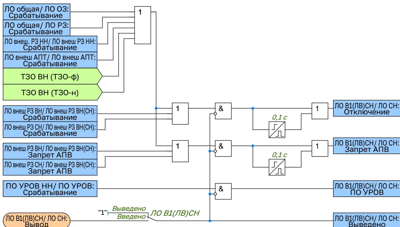
Рисунок 2.42 – Функциональная схема логики отключения V1(ЛВ) СН
