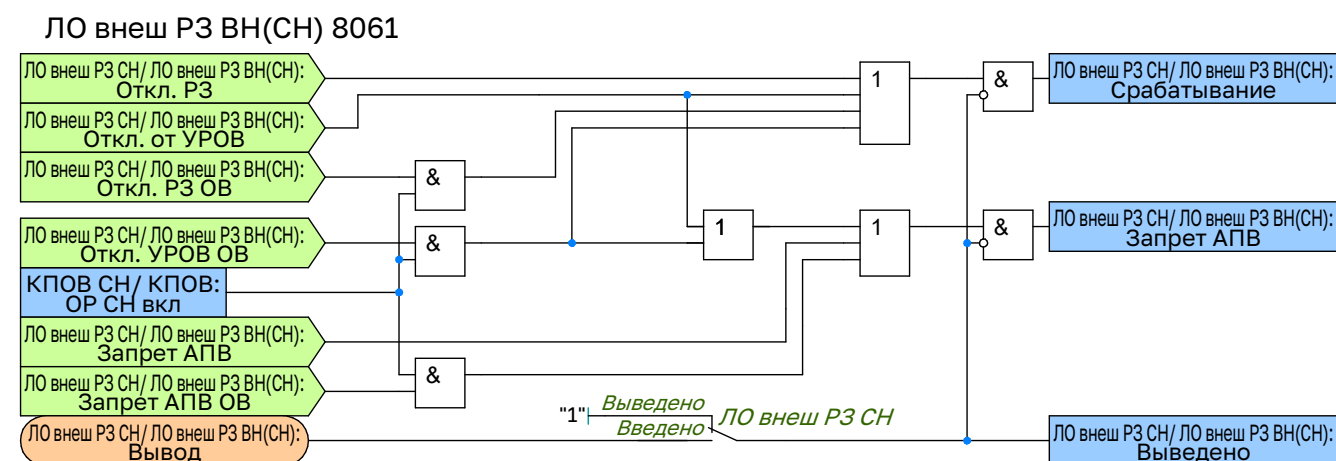
Рисунок 2.37 – Функциональная схема логики внешних отключений СН
