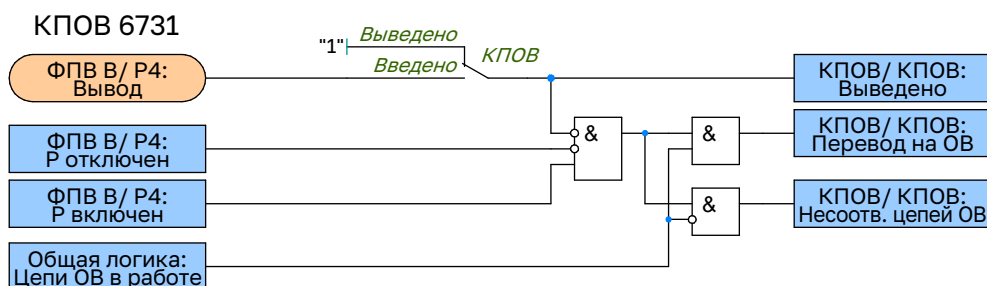
Рисунок 2.46 – Функциональная схема логики контроля перевода на ОВ
